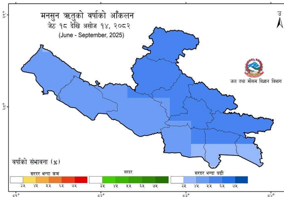
चित्र २: २०८२ मा लुम्बिनी प्रदेशमा वर्षाको आँकलन
