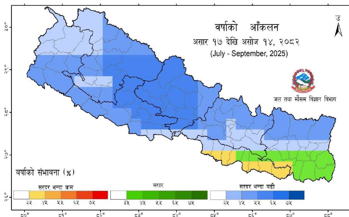
चित्र-१: २०८२ मनसुनमा नेपालभर वर्षाको आँकलन
